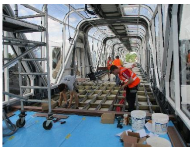
Installation du platelage
