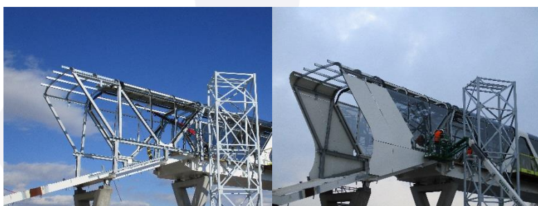
Mise en place progressive de la couverture
